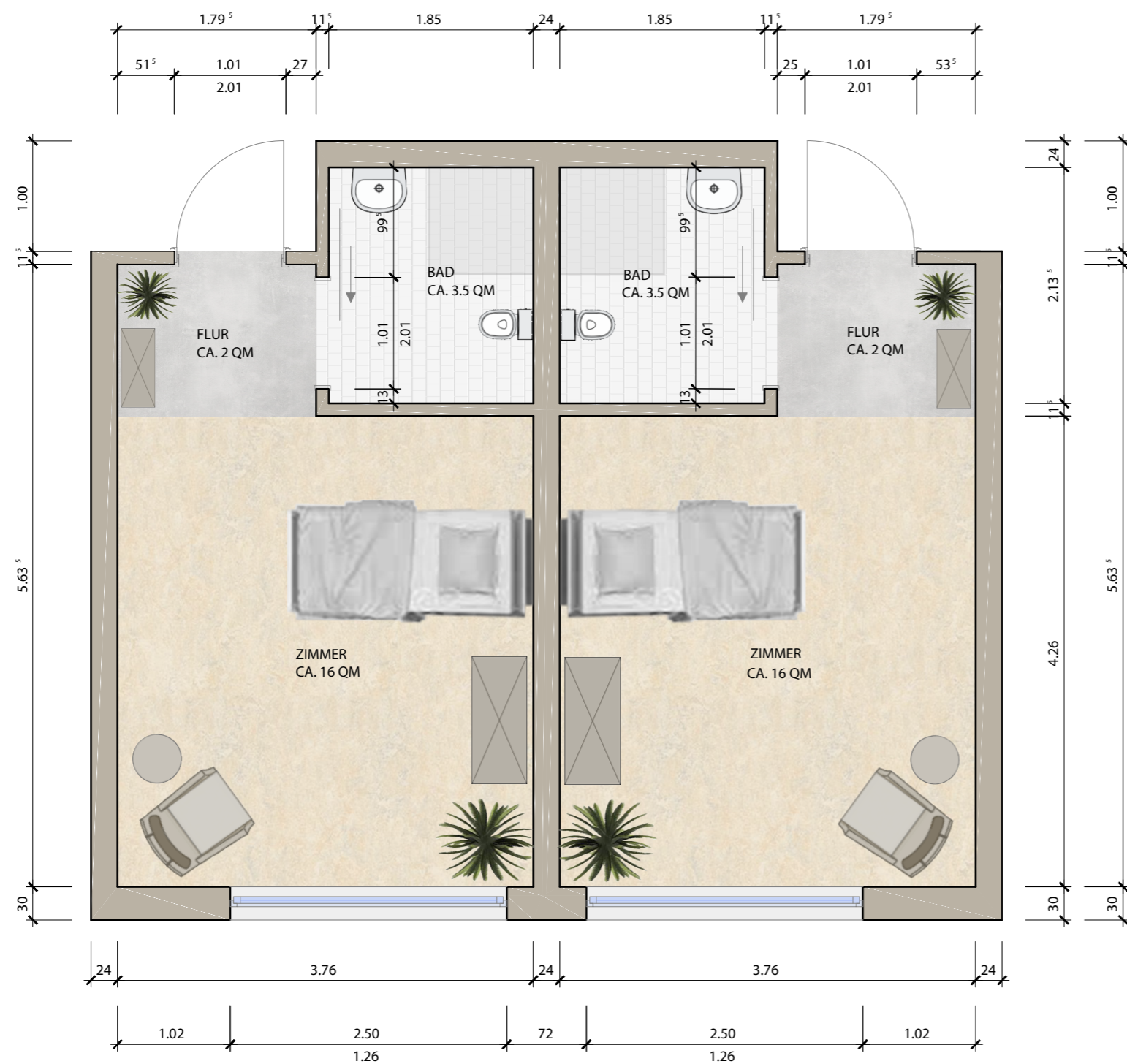
EINBETTZIMMER BAUTEIL C 2. OG - WEILBACH
